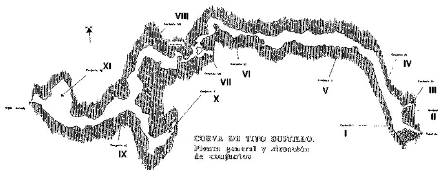
Plano general de la cueva de Tito Bustillo
